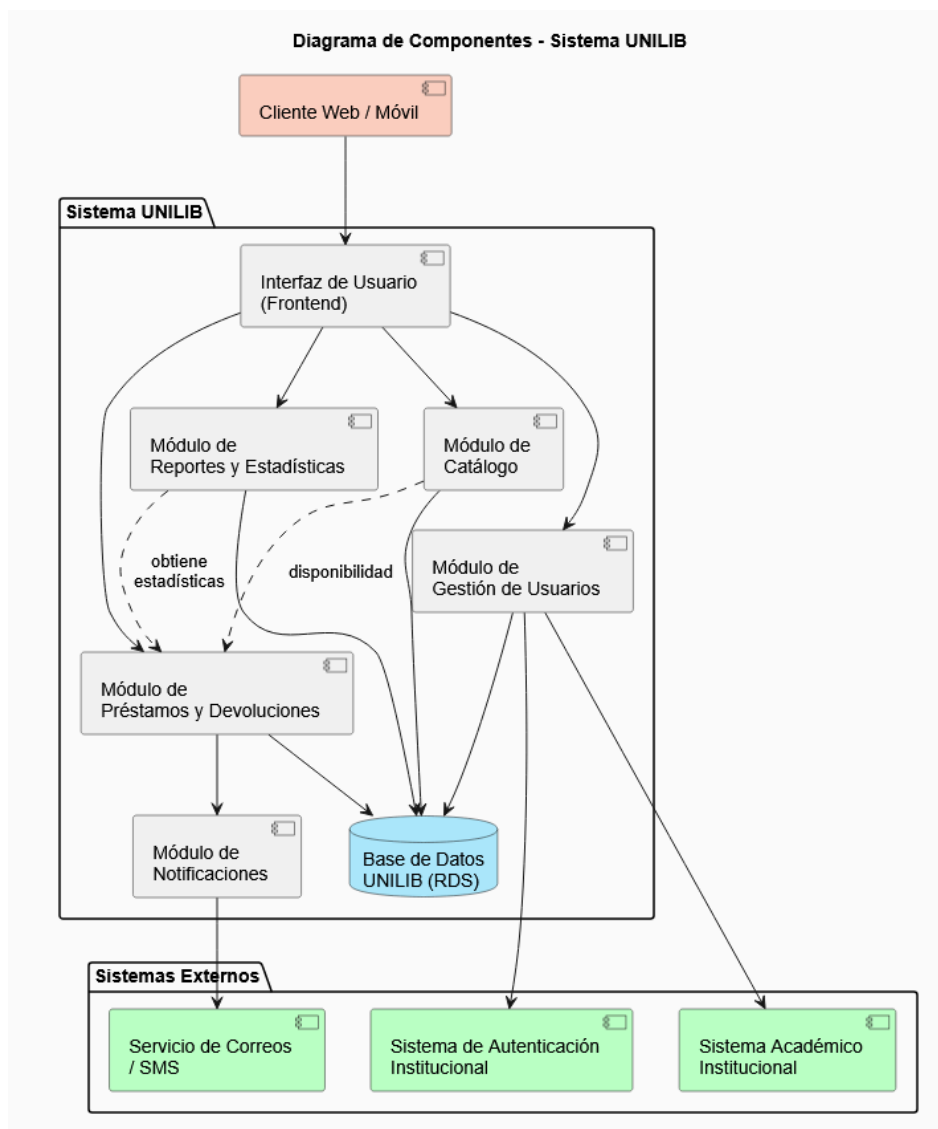
Ilustración 4: Diagrama de Componentes
