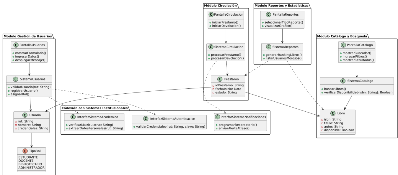
Ilustración 1: Diagrama de Clases
